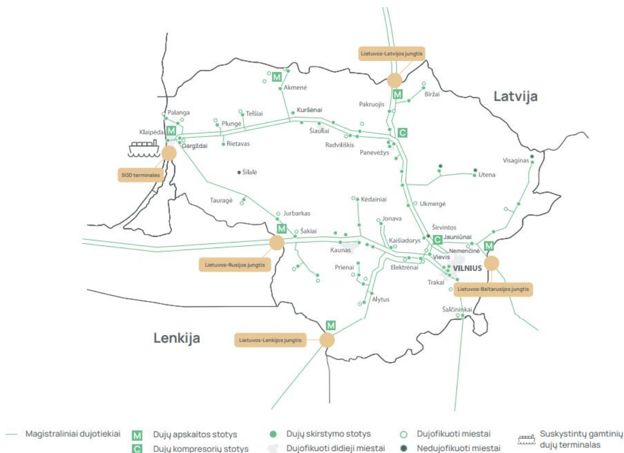
12.2.Pav. Pagrindinis ir lokalus gamtinių dujų perdavimo tinklas, 2022 m. 2
