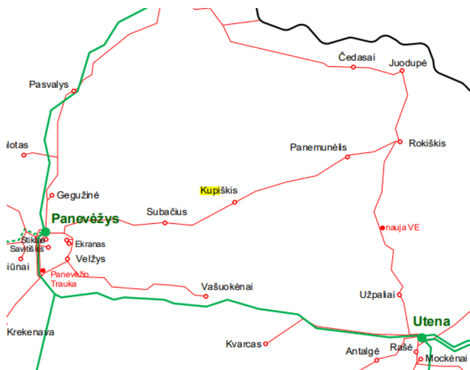
12.1. Pav. Lietuvos EES 400-110 kV perdavimo tinklų schemos ištrauka
